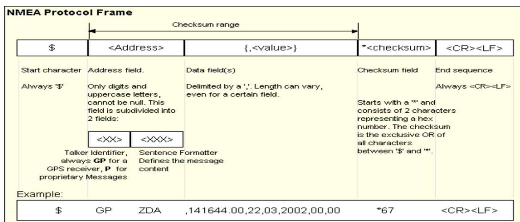
그림 11. NMEA 프로토콜 프레임
