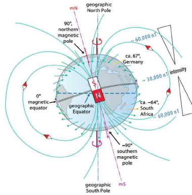
그림 14. 자북과 진북 비교
